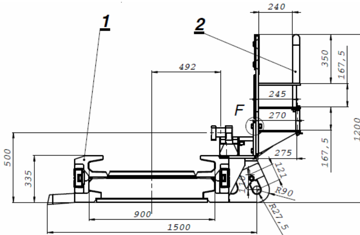
Przekrój trasy przenośnika PSZ 950 Nowomag
