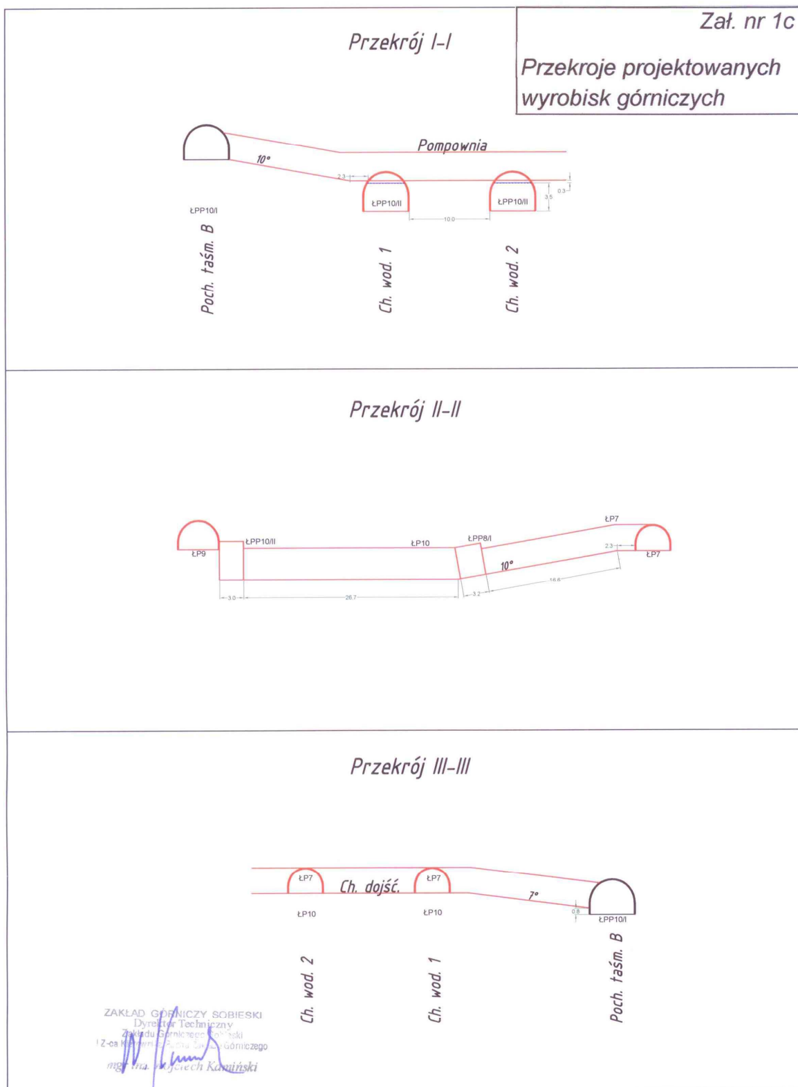
Chodniki odwodnienia lokalnego, komora pomp w rejonie pochylni taśmowej B -przekroje
