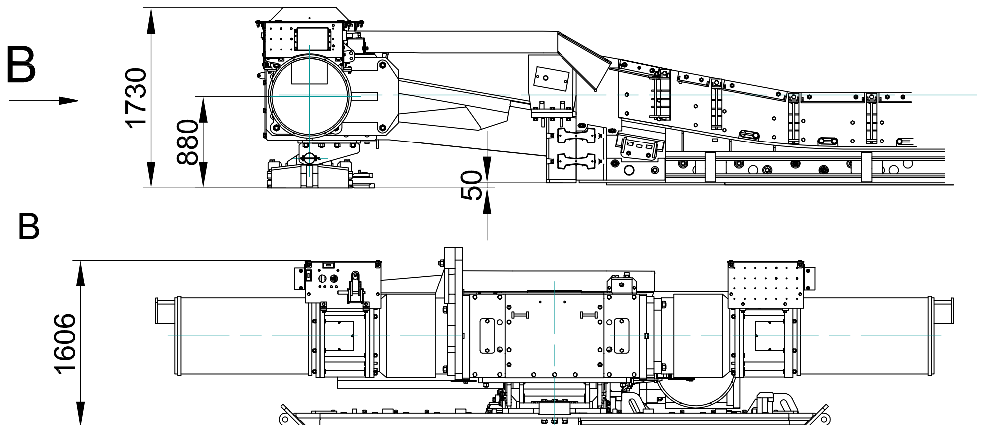
Napęd wysypowy przenośnika Glinik 298/800/BP w przypadku zastosowania jednostek prostopadłych
